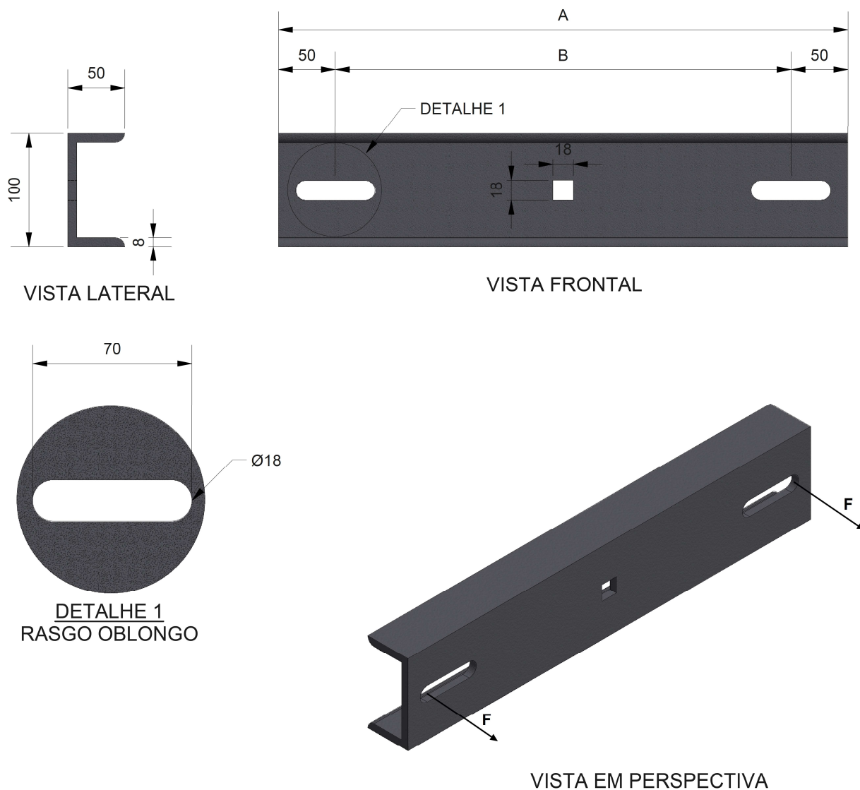
Figura 4 - Cantoneira "U" tipo 4
