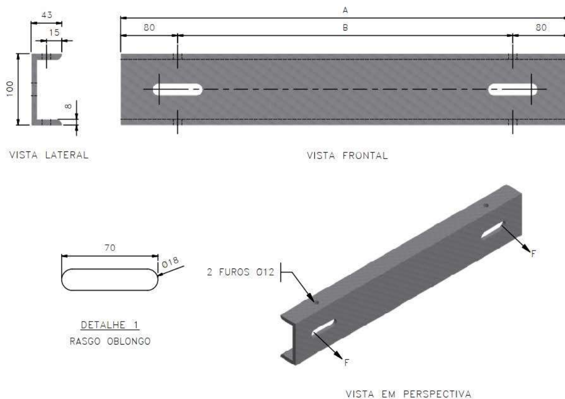
Figura 2 - Cantoneira "U" tipo 2
