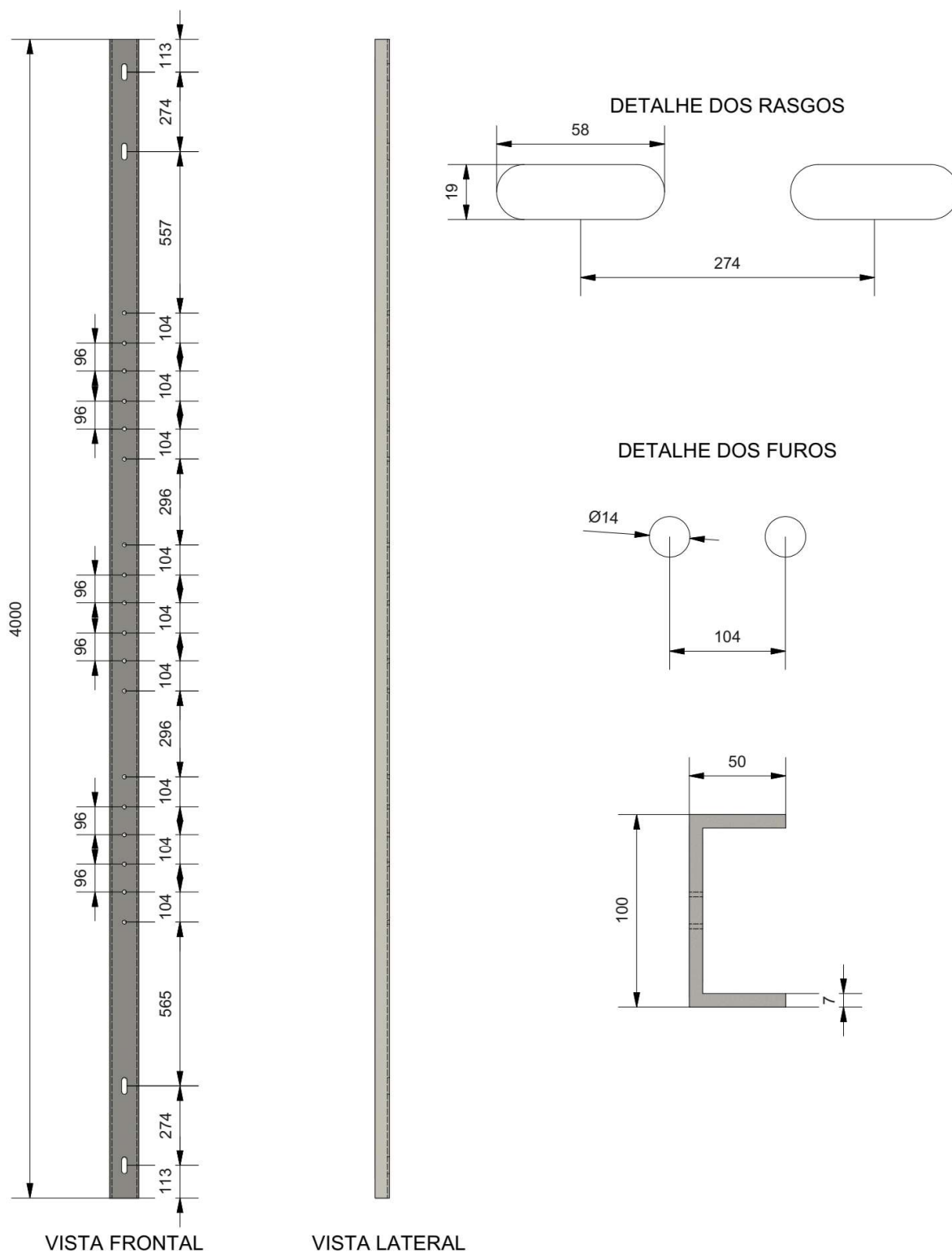
Figura 6 - Cantoneira "U" tipo 6
